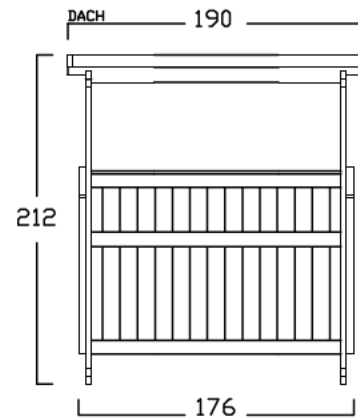
AUSSENWAND
