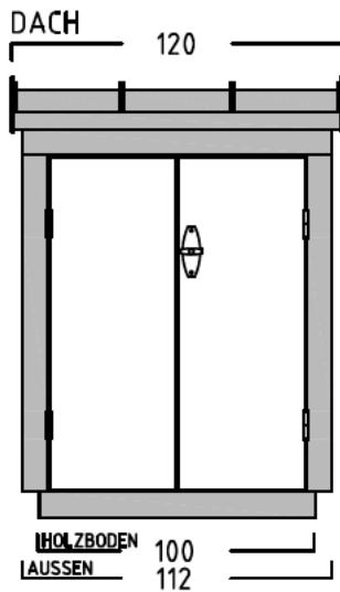
ANSICHT: EINFAHRWAND
