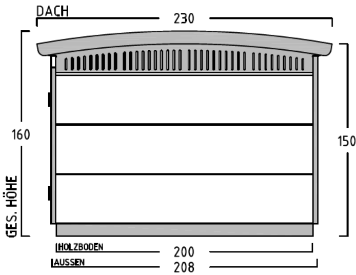
ANSICHT: RECHTE SEITENWAND
