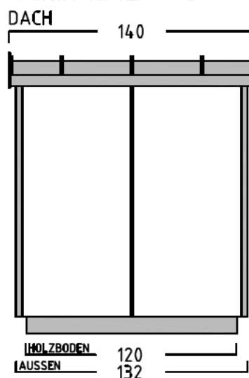
ANSICHT: HINTERWAND
