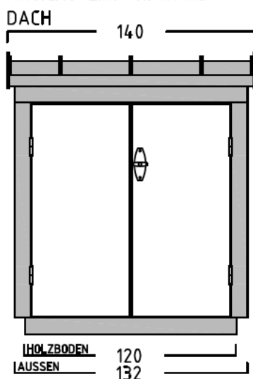
ANSICHT: EINFAHRWAND
