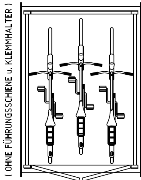
FAHRRADAUFNAHME 2 bis 3
